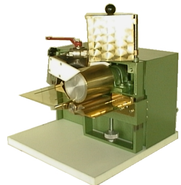
Edge Top Glue roller Mod. Mercur 90 mm
